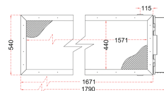
вид сзади
