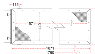
вид спереди
