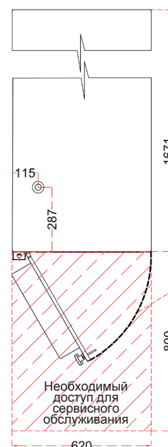
вид сверху
